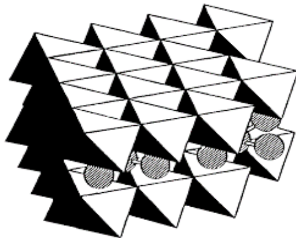
Figura 1. Estrutura da hidrotalcita ( [Mg_6Al_2(OH)_{16}]CO_3 \cdot 4H_2O ).
