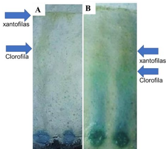
Figura 3: Cromatografia em camada delgada de extratos de sara-tudo. (A) Placa cromatográfica com acetona como fase móvel. (B) Placa cromatográfica utilizando a mistura de acetona e removedor de gordura como fase móvel.
