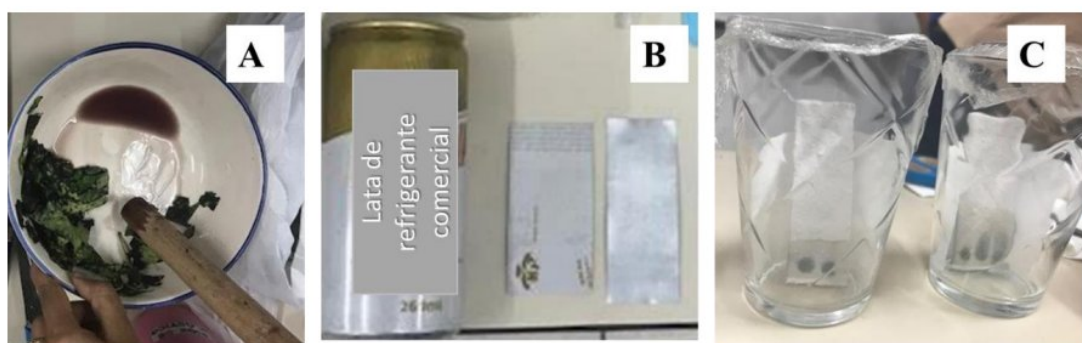
Figura 2: Preparação das placas cromatográficas. A) Extração; B) preparação dos suportes; C) eluição. Fonte: Os autores, 2020.
