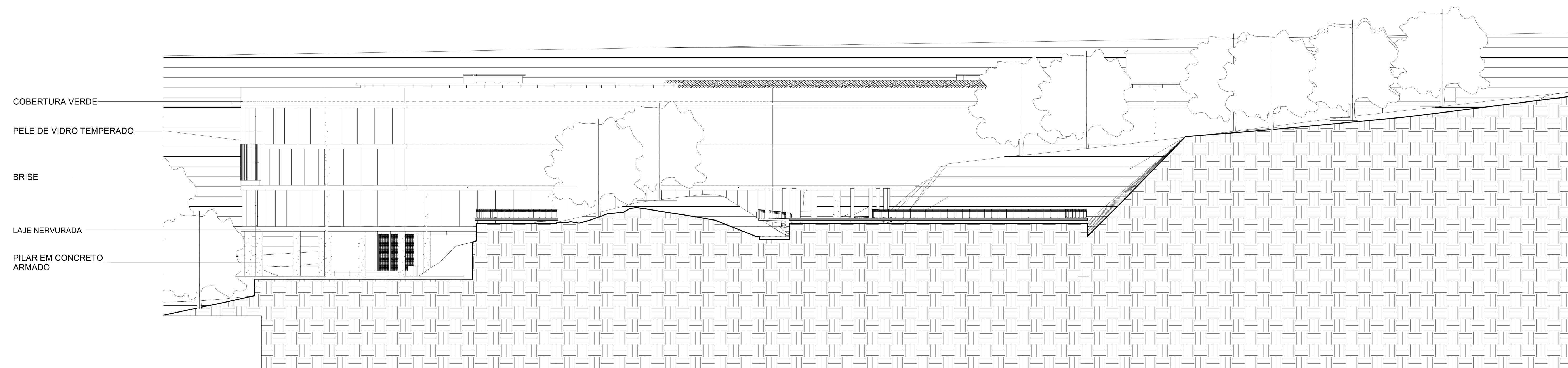
5 Sul 1 : 200
