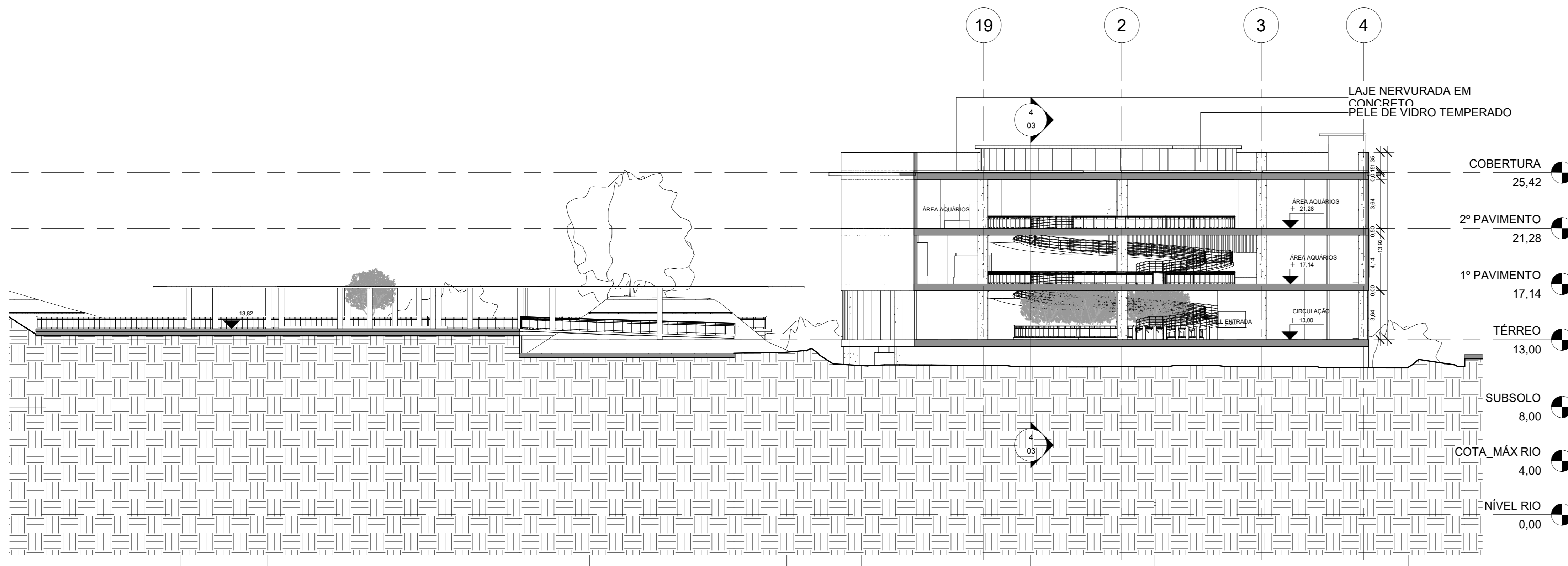
1 Corte AA' 1 : 200
