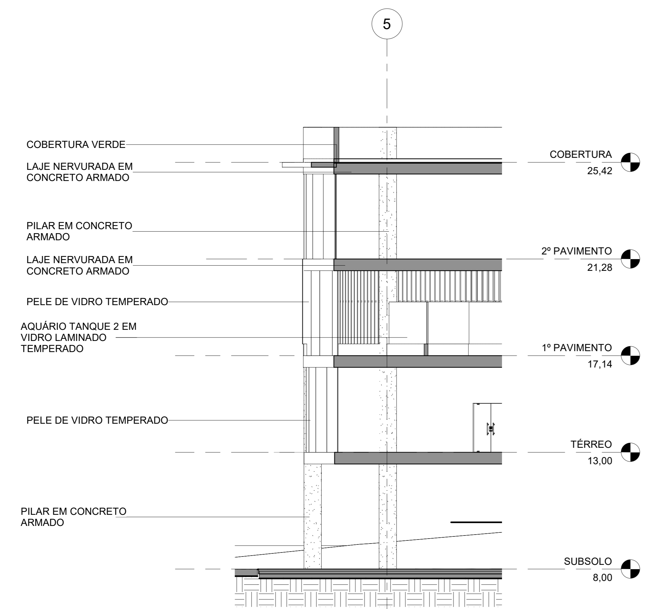
4 Corte 0 1 : 100
